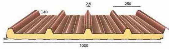
Pannello coibentato grecato
